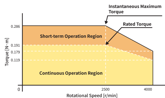
EzPM-G-GMX200AD
