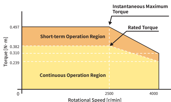
EzPM-G-GMX100AD
