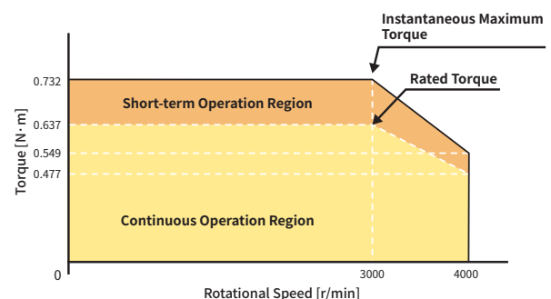
EzPM-G-GMX200AD
