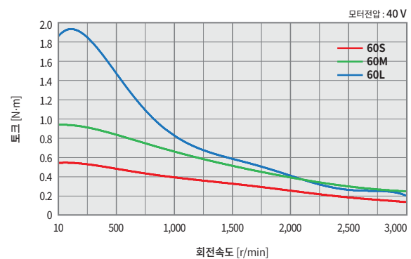
Ezi-SERVO-CT-60 타입
