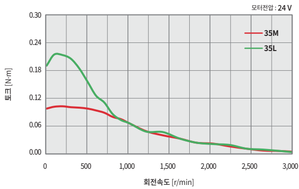
Ezi-SERVO-CT-4X-HSP35 타입
