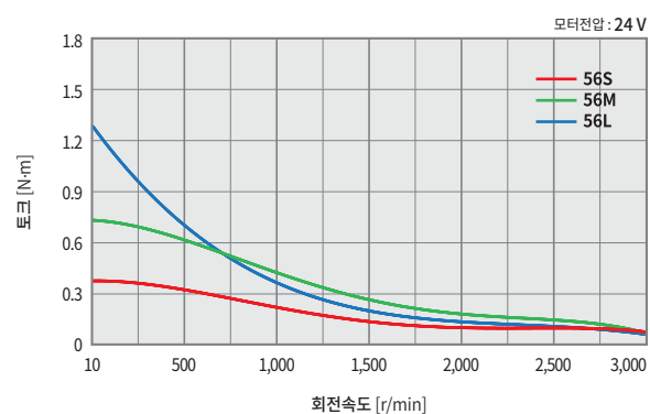
Ezi-SERVO-CT-4X-56 타입
