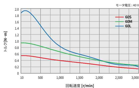
Ezi-SERVO-CT-60 シリーズ
