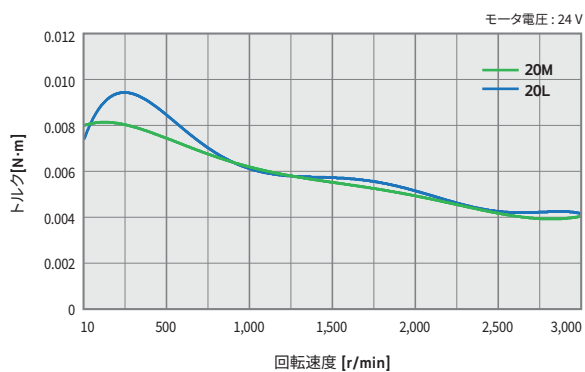
Ezi-SERVO-CT-35 シリーズ
