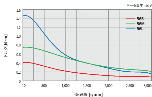
Ezi-SERVO-CT-56 シリーズ
