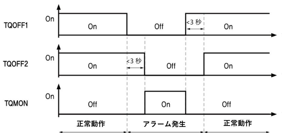
<TQOFF入力（正常動作）>
