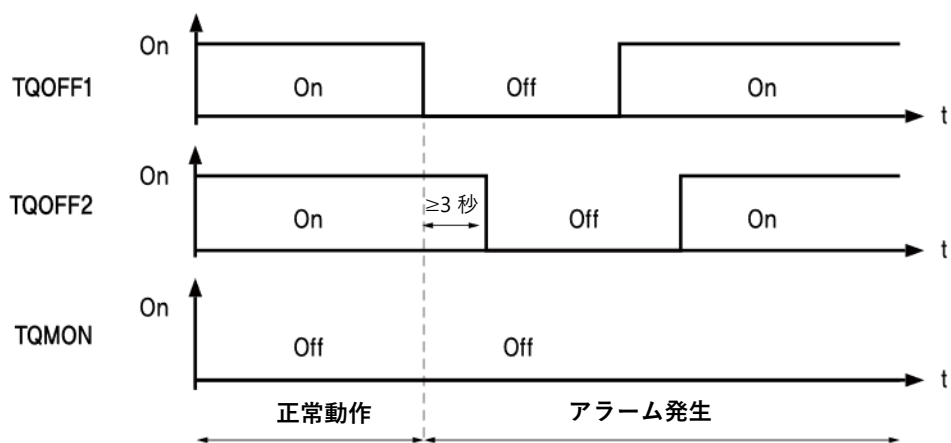
<TQOFF入力（異常動作）>
