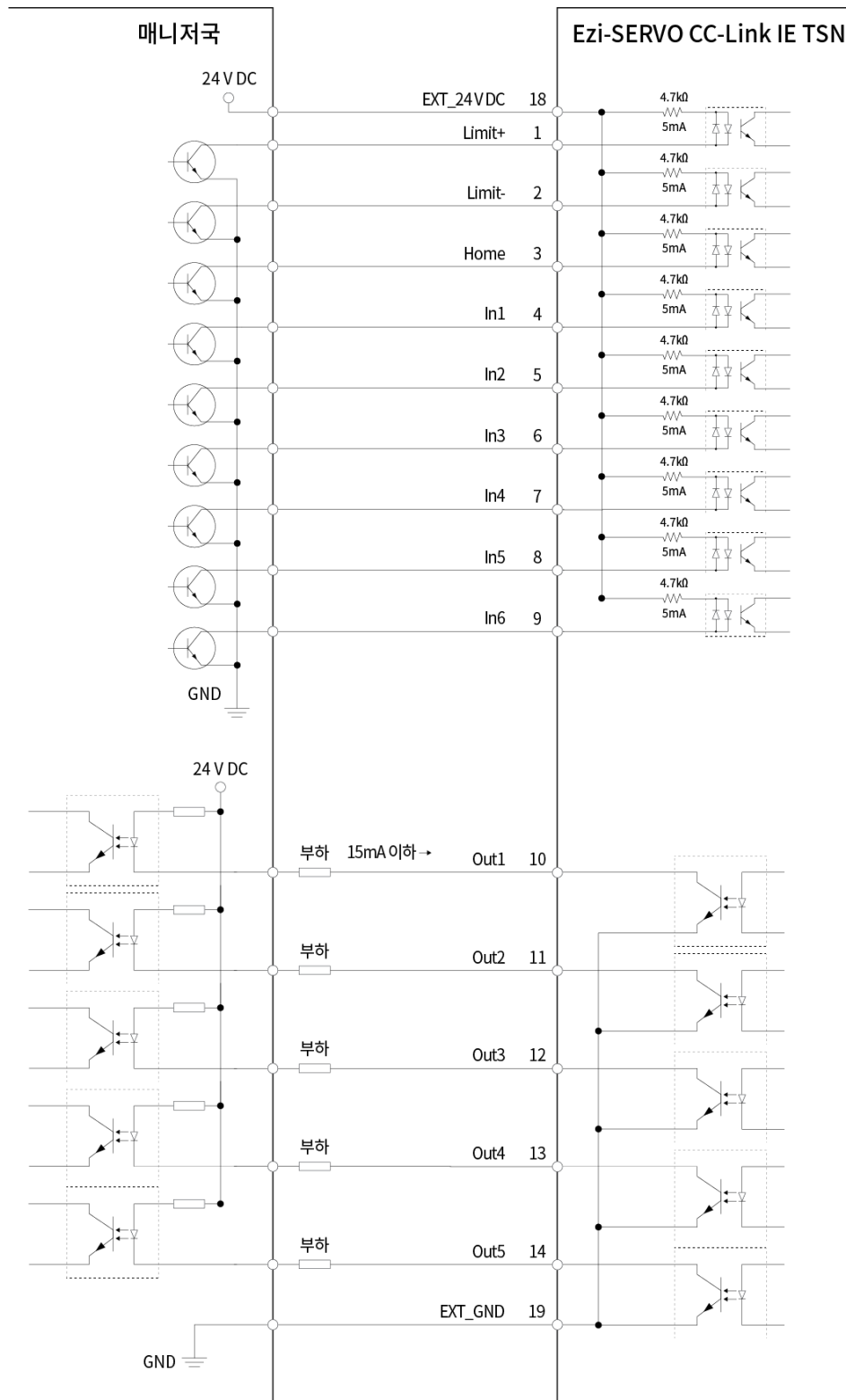
(f) 전류 싱크 출력회로와 접속하는 경우
