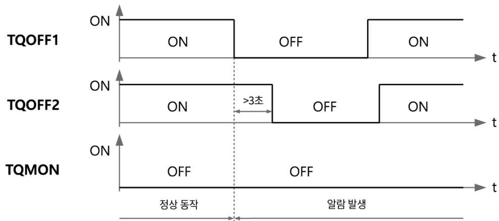
&lt;TQOFF 입력 (비정상 동작)&gt;
