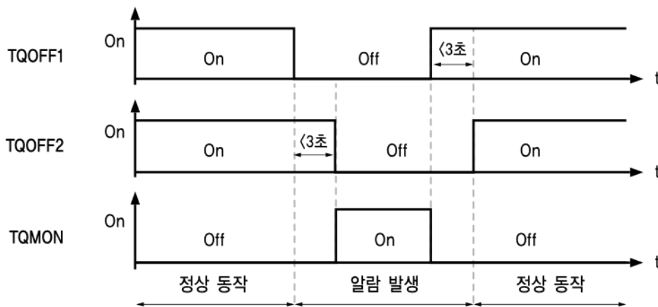
<TQOFF 입력 (정상 동작)>
